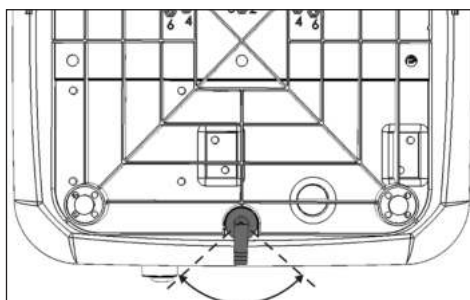
Orientation de l'évacuation des condensats (vue du dessous de l'appareil)
